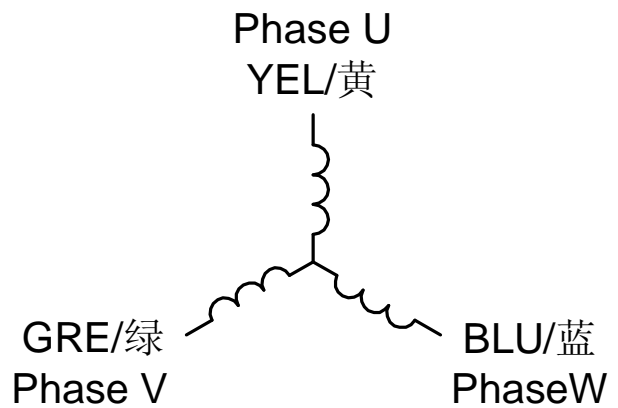
绕组接线图 Winding Diagram
