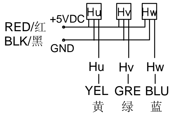
霍尔接线图 Hall Sensor Wiring Diagram
