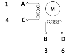
励磁顺序vs.旋转方向
