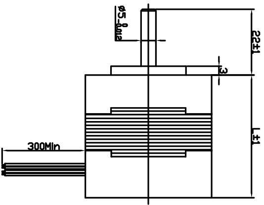
电机外形尺寸图 Motor Dimension (mm)
